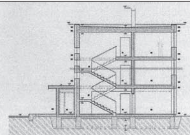
rez - alternatíva s plochou strechou
