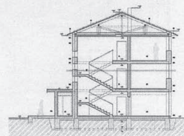
rez - alternatíva so sedlovou strechou (podkrovia bez účelu)
